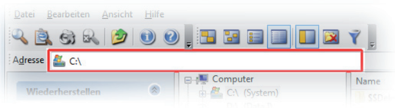
Schnellsuche
